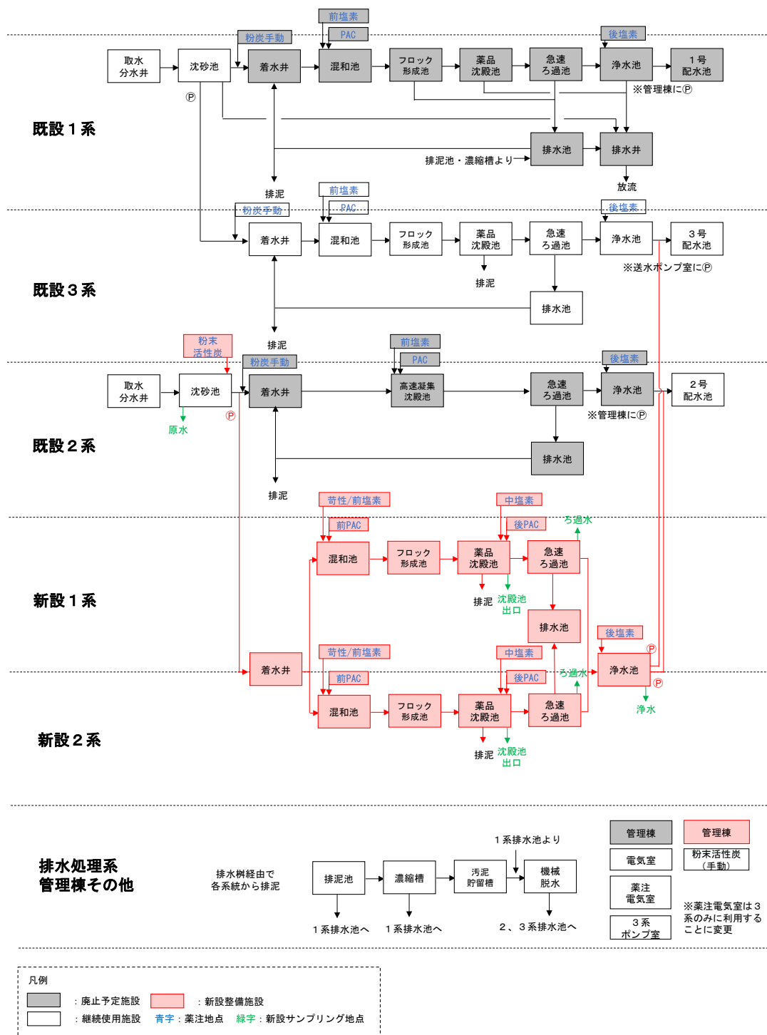
図 2-2 更新前後の施設フロー
