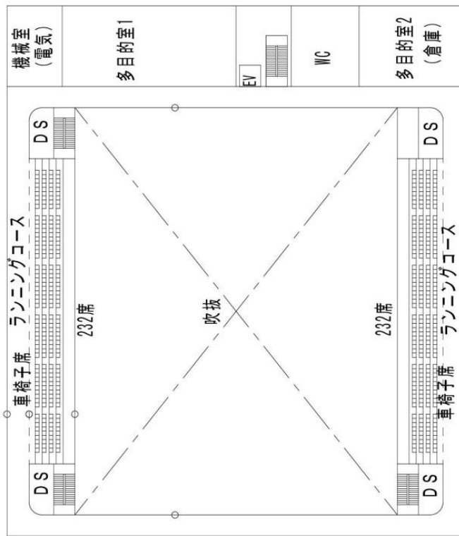
2階平面図
