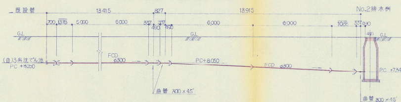
③ 縦断展開図 S=1/100
