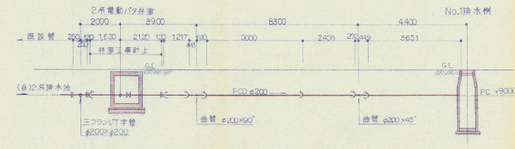
④ 縦断展開図 S=1/100
