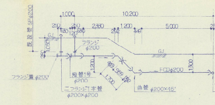
⑥ 縦断展開図 S=1/100
