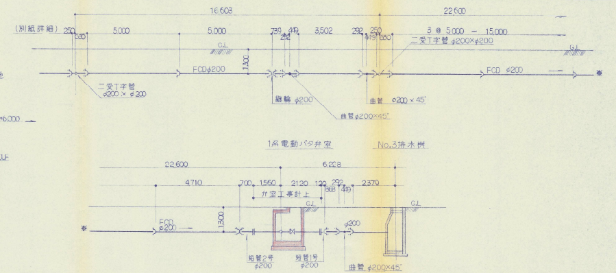
⑤ 縦断展開図 S=1/100
