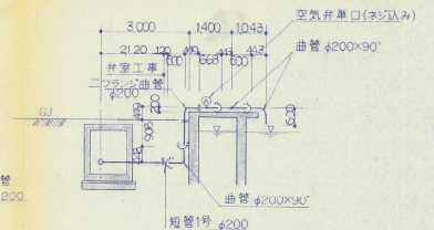
⑦ 縦断展開図 S=1/100
