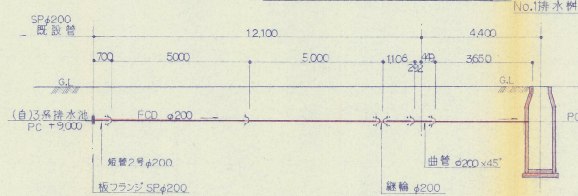
③ 縦断展開図 S=1/100
