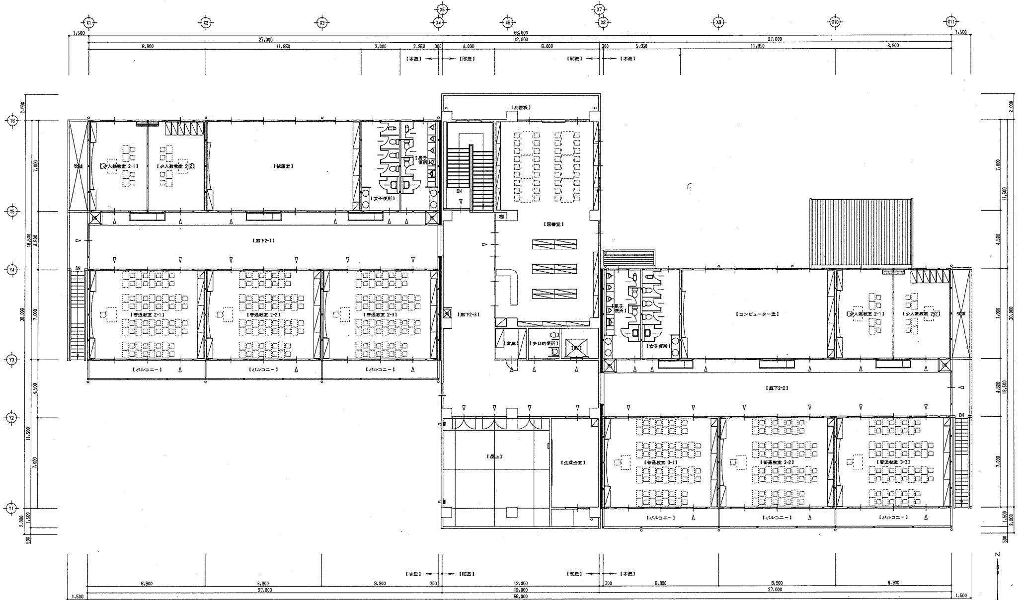
2階平面図
