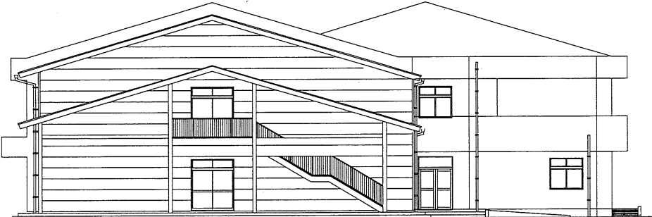
西側立面図
